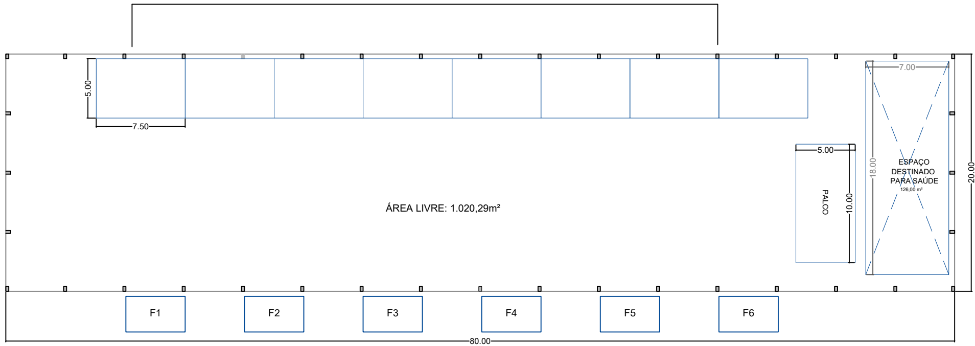
PLANTA BAIXA PRAÇA DE ALIMENTAÇÃO ÁREA TOTAL: 1.600,00 m²
