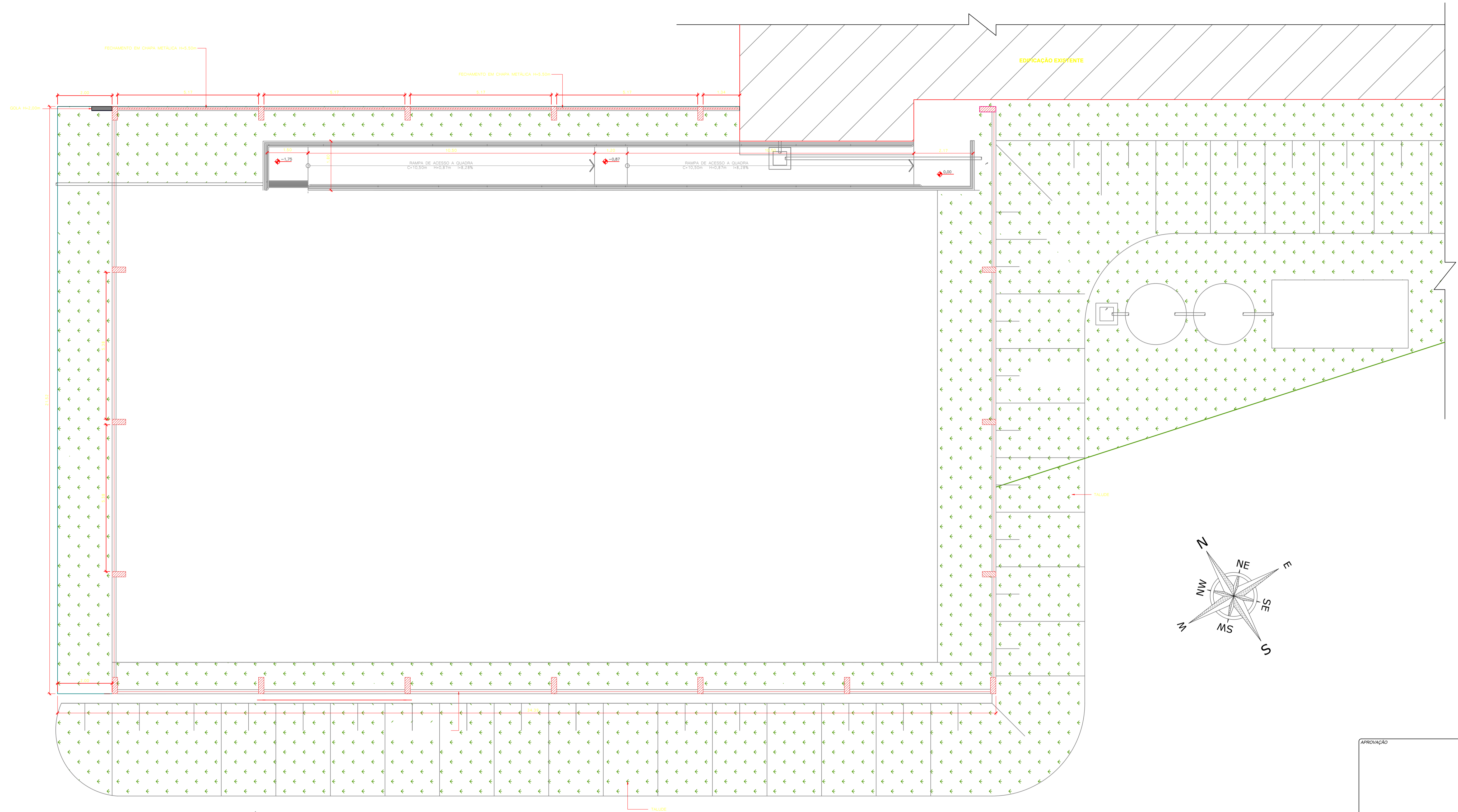
PLANTA BAIXA ESC: 1/50
